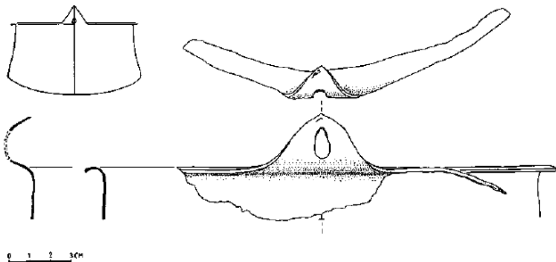
Fig. 2; Nederwetten 1989, Randfragment van de koperen ketel van het 'Vestlandtype'.
